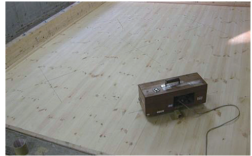
軽量床衝撃音試験 (タッピングマシン)
